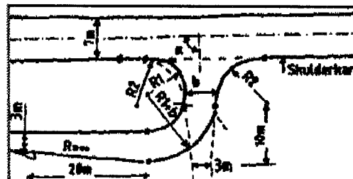
Når kryssvinkel er 90^\circ < \alpha < 100^\circ , nyttast stipla utforming Utforming av avkjørsler
