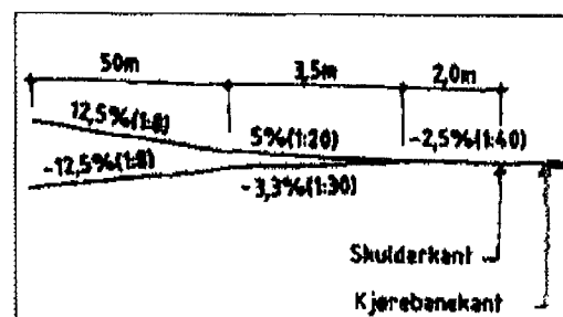
Lengdeprofil av avkjørsel, grenseverdier.
